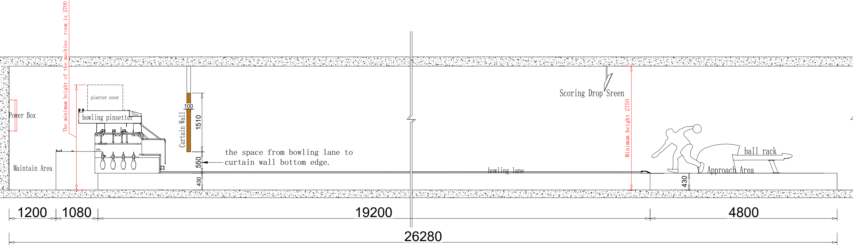
ELEVATION
